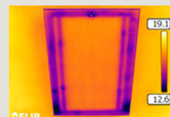
Традиционная лестница с утеплением 70 см - большие потери тепла по периметру.
